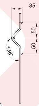
Gradil Elevação esc. 1:35
