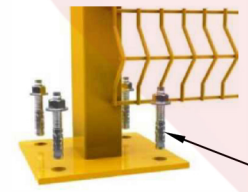
Parabolt tipo PBA 3/8 X 3"
